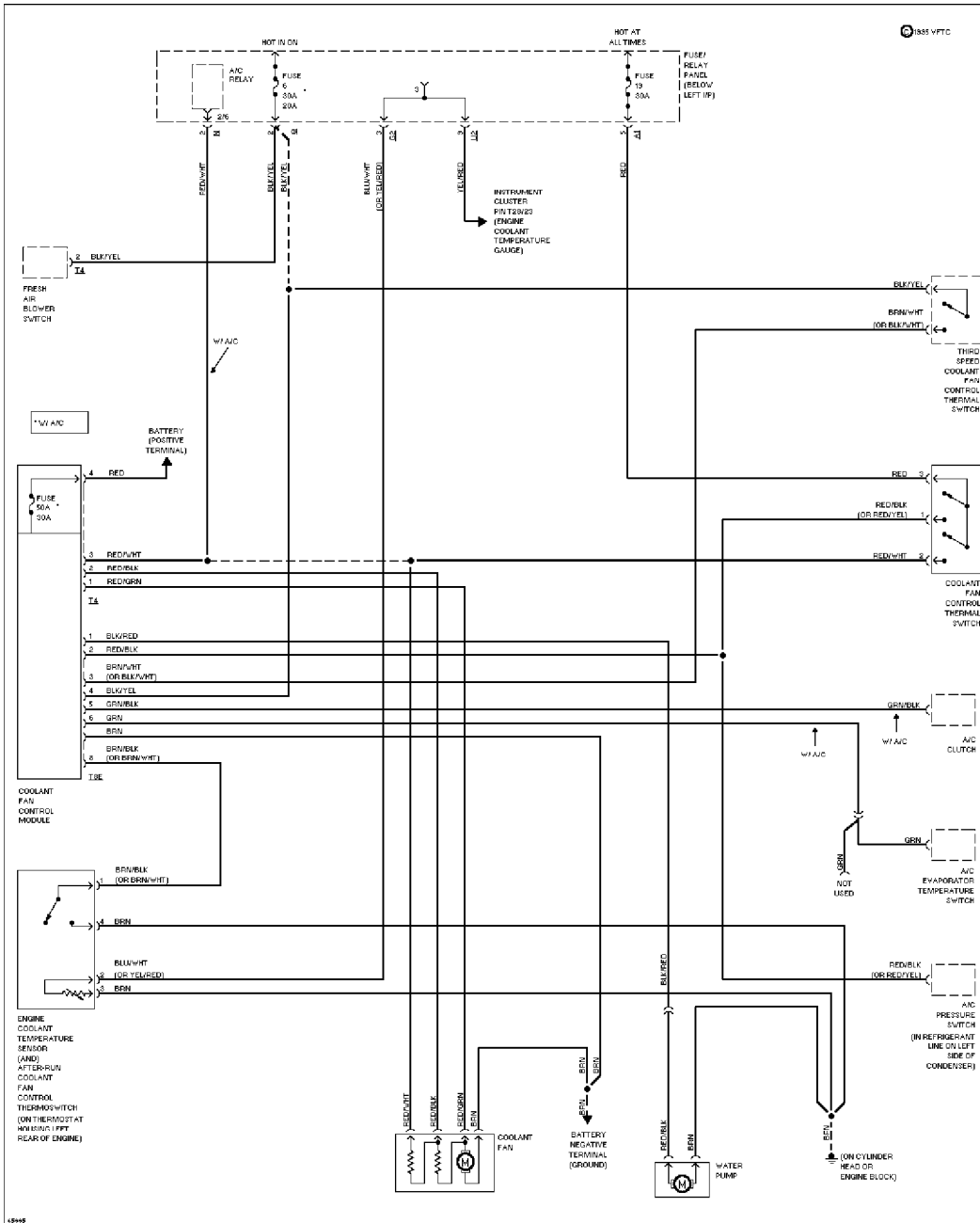
48998 Cooling Fan Circuit
